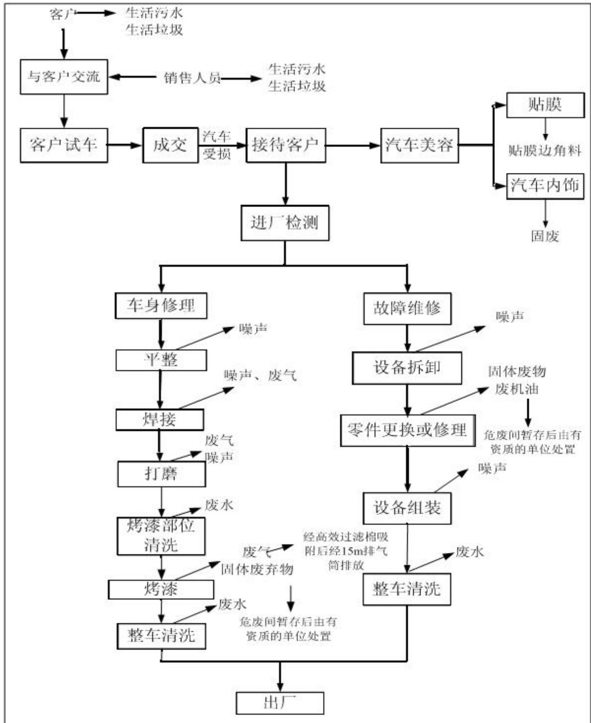
图 2.2-1 项目工艺流程及产污环节图
