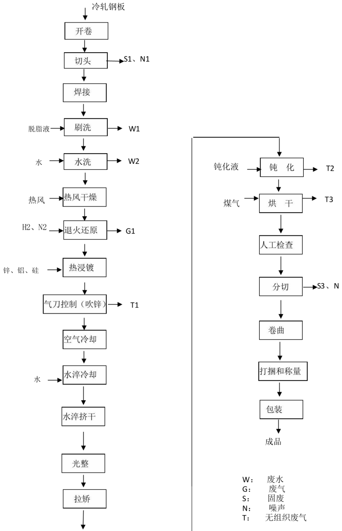
图 2.2-1 热镀铝锌硅钢板生产工艺流程图
