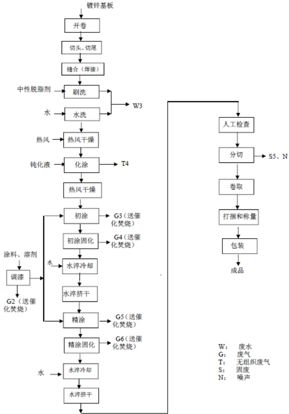
图 2.2-2 彩涂板生产工艺流程图
