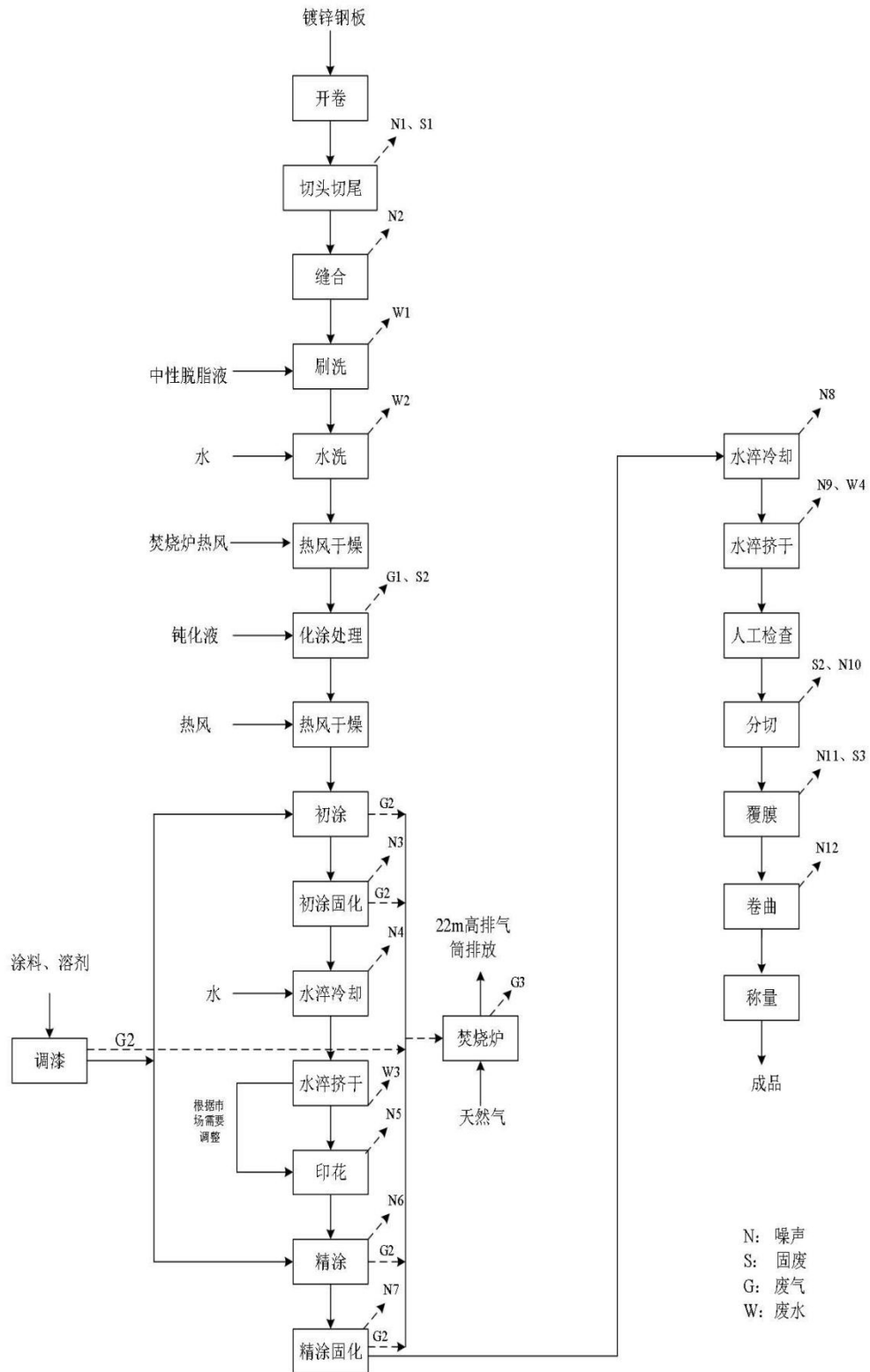
图 3.4-3 彩涂印花钢板生产工艺流程及产污环节
