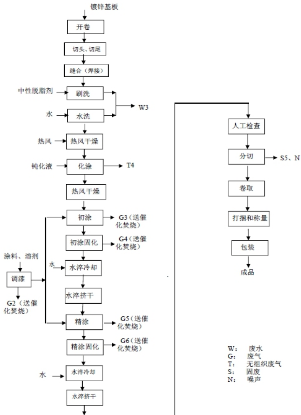
图 3.4-2 彩涂板生产工艺流程图
