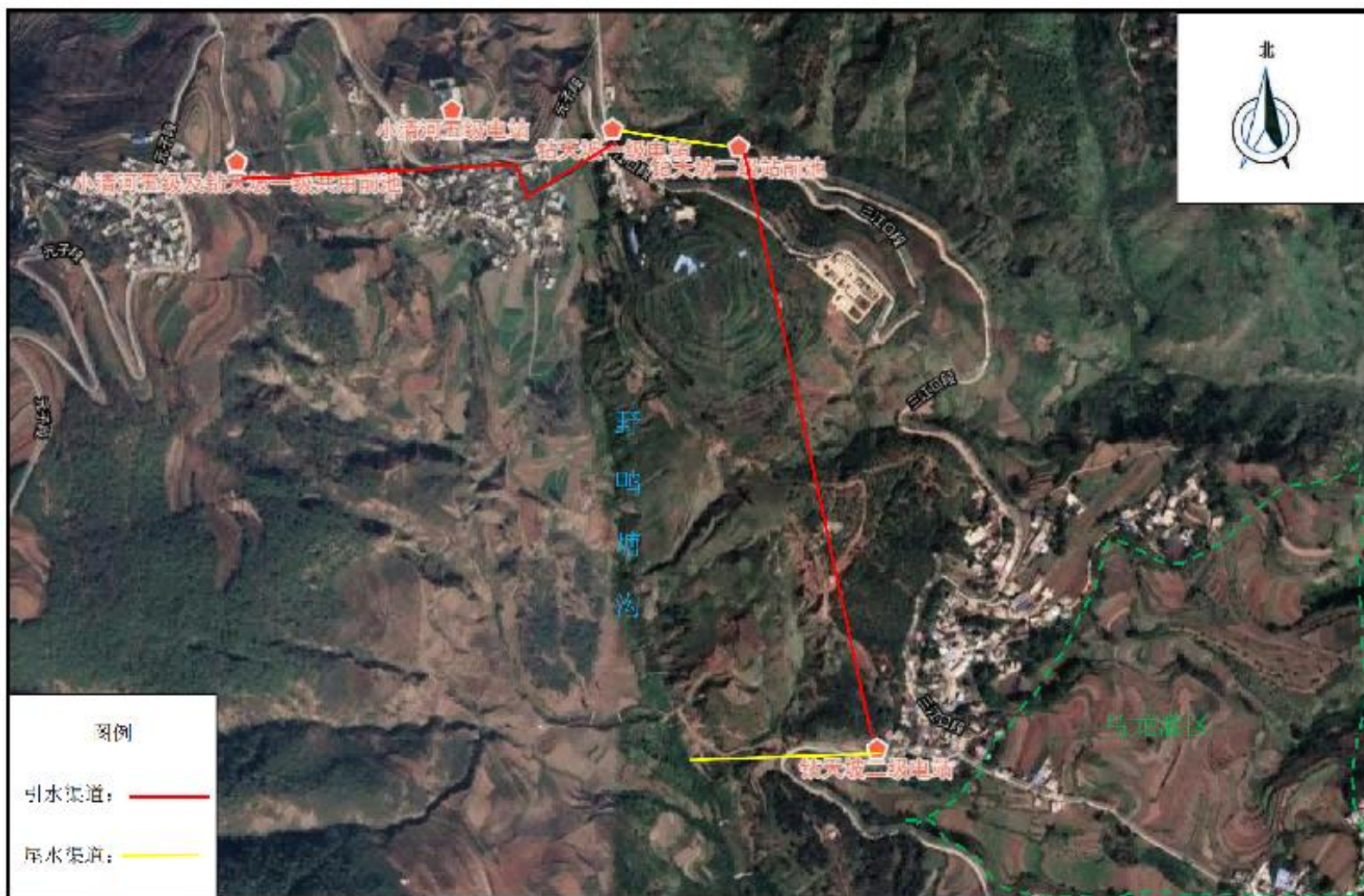
附图5 建设项目来水、尾水渠道走向布置示意图
