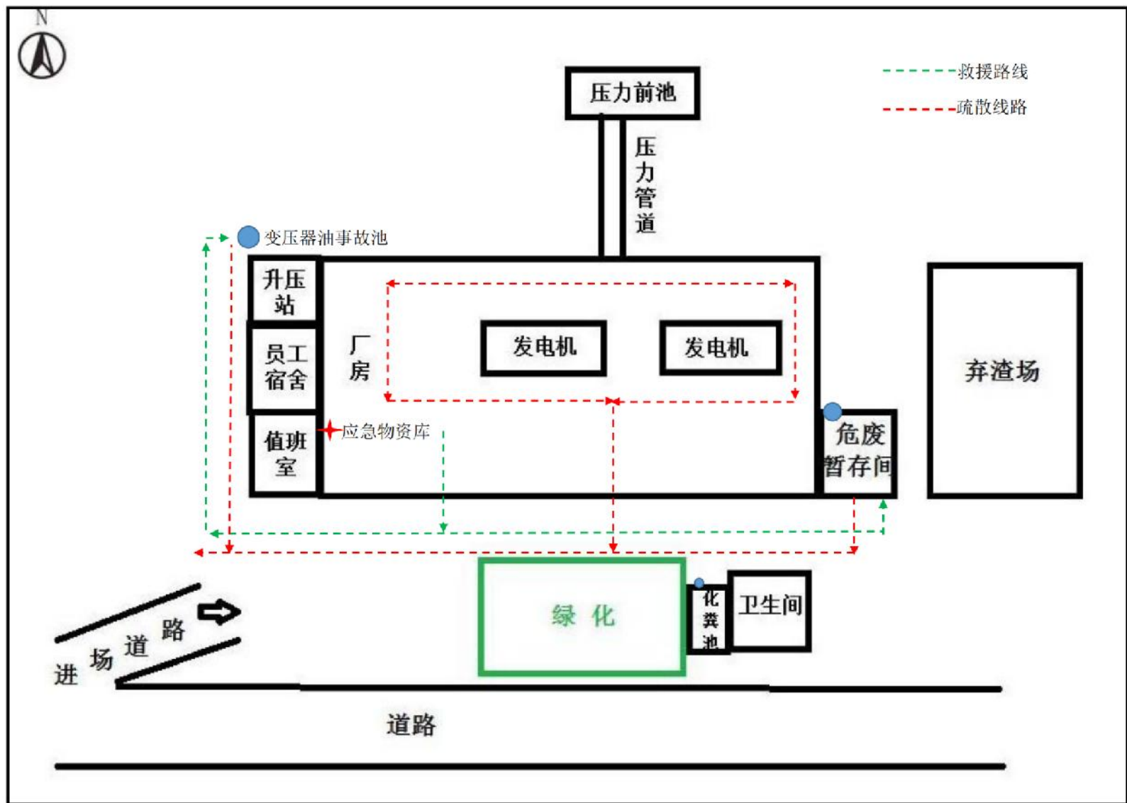
附图 4 钻天坡二级平面布置、应急物资分布及疏散路线图
