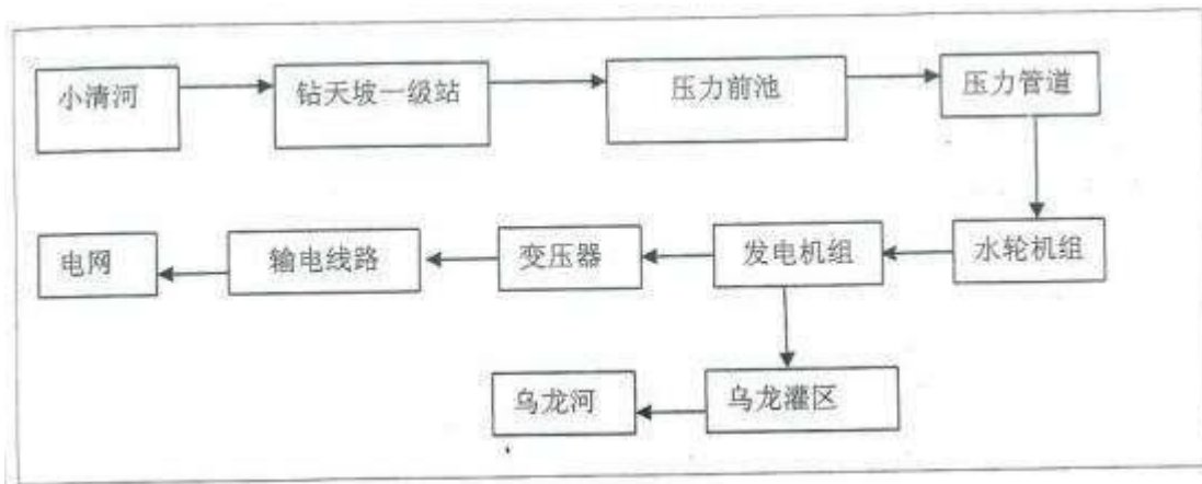
图 2.2-1 钻天坡二级电站生产工艺流程图
