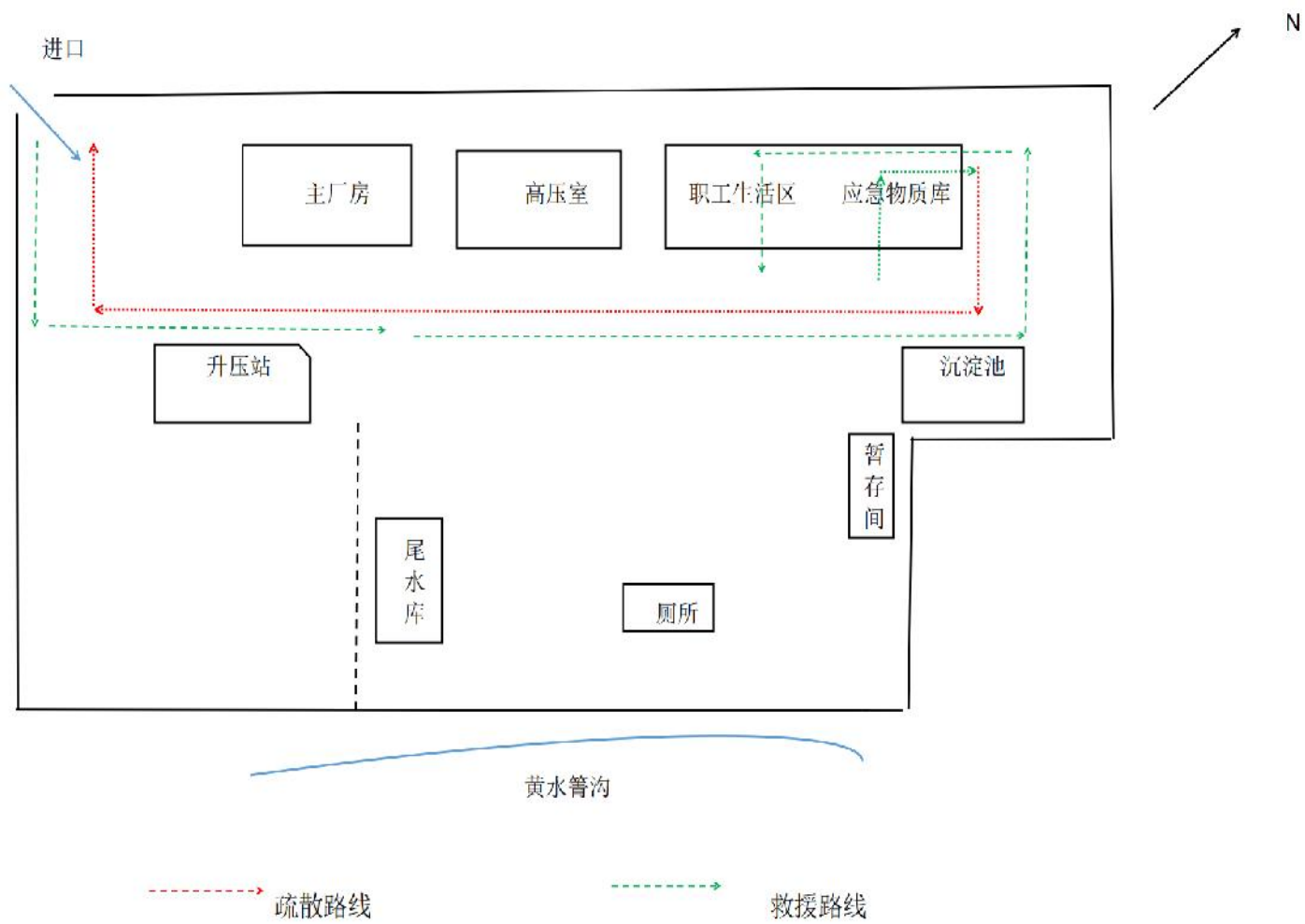
附图 4-2 建设项目平面布置、环境风险源位置及疏散线路图
