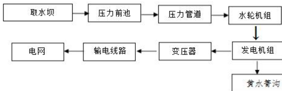
图 2.2-1 昆明市秀水河电力有限公司生产工艺流程图
