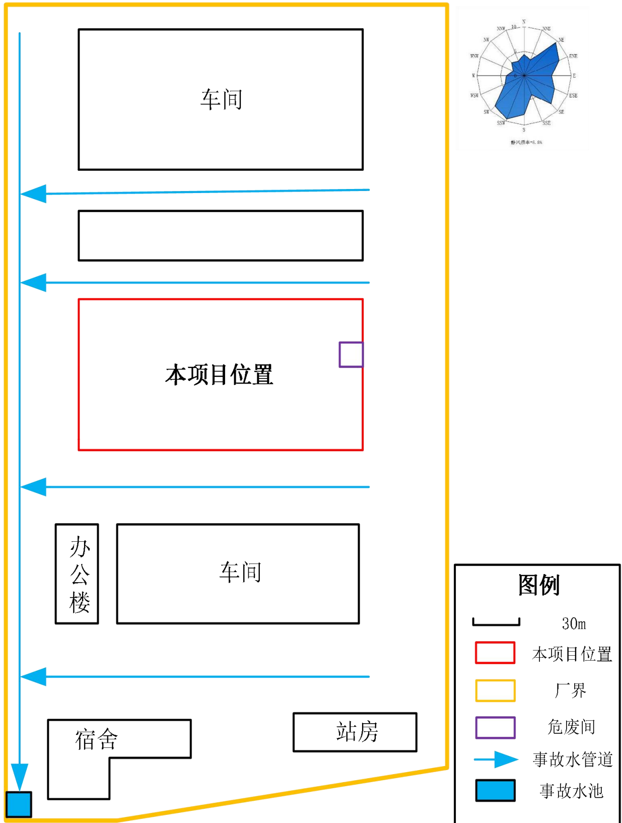
附图3-1 项目厂区平面布置图
