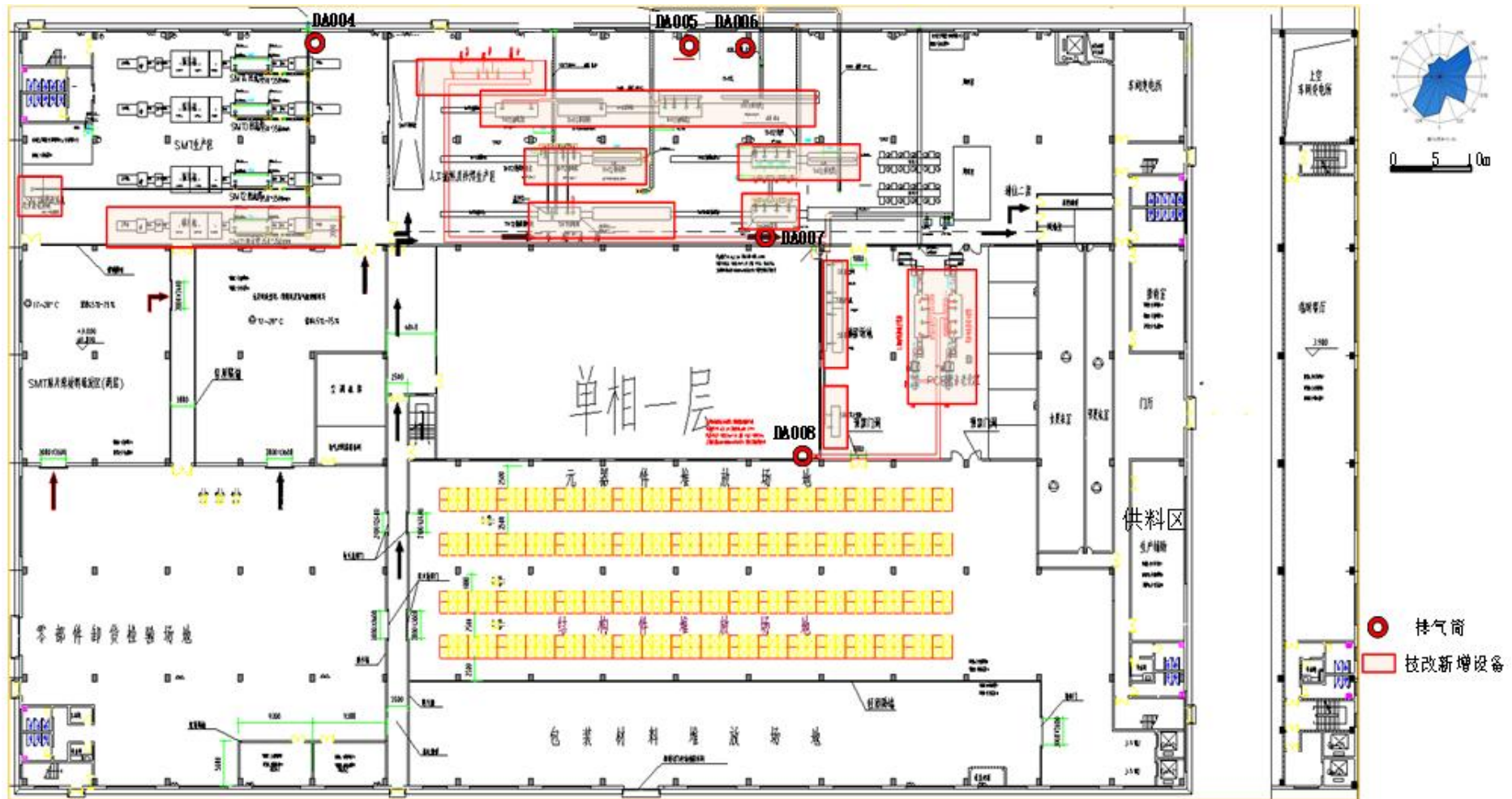
附图3-2 项目车间1F平面布置图
