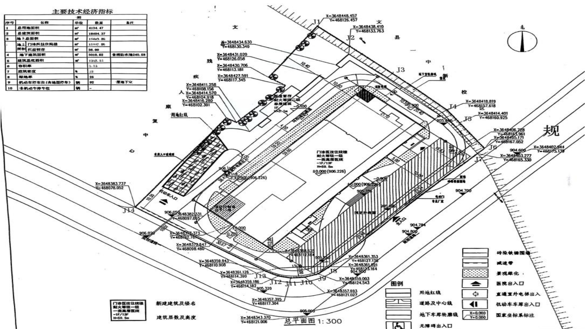
图3 总平面布置图
