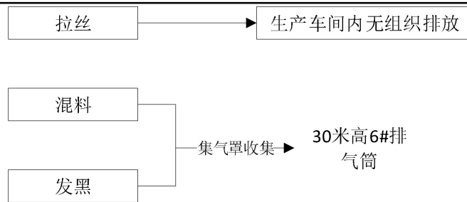
图 4-1 废气走向图
