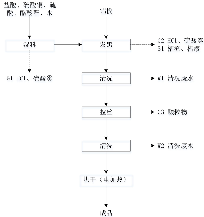
图2-3 发黑线生产工艺及产污节点图
