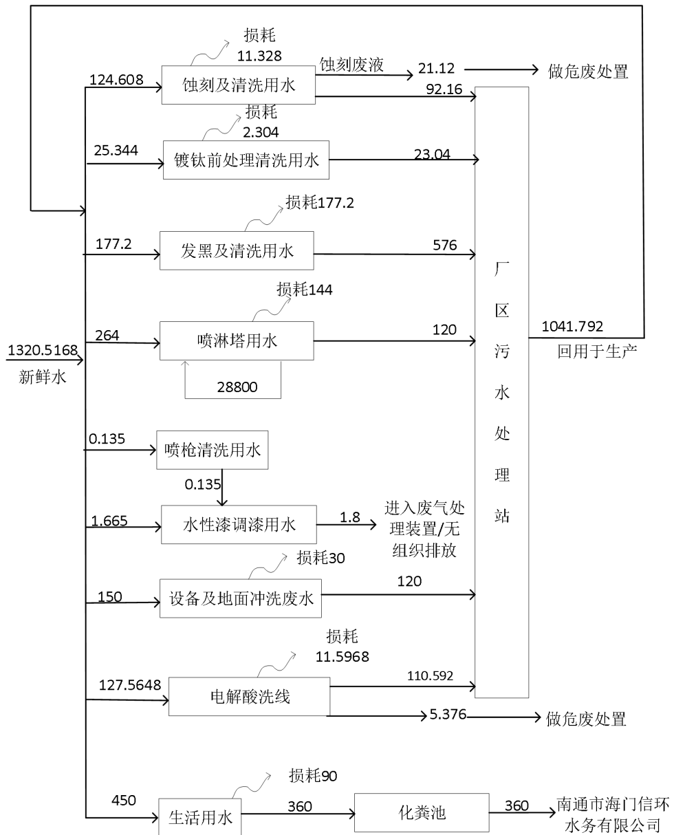
图2-1 (2) 本项目建成后全厂水平衡图 (m³/a)
