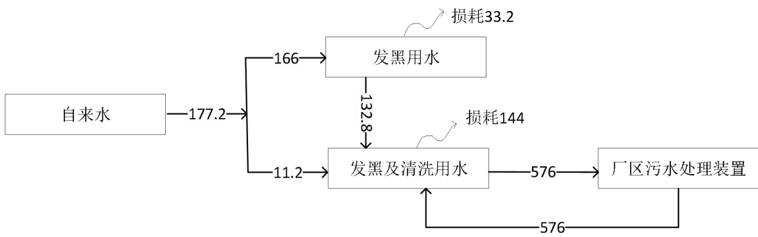
图2-1 (1) 本项目水平衡图 (m³/a)
