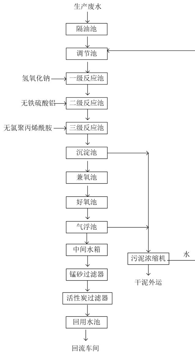
图 4-3 综合废水处理工艺流程
