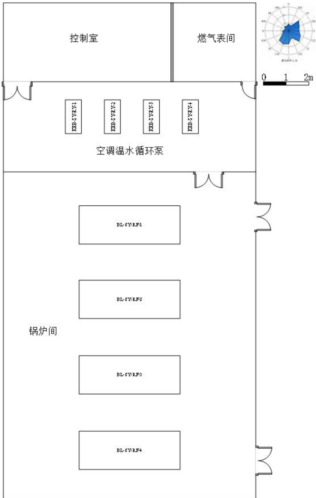
附图3-2 锅炉房平面布置图
