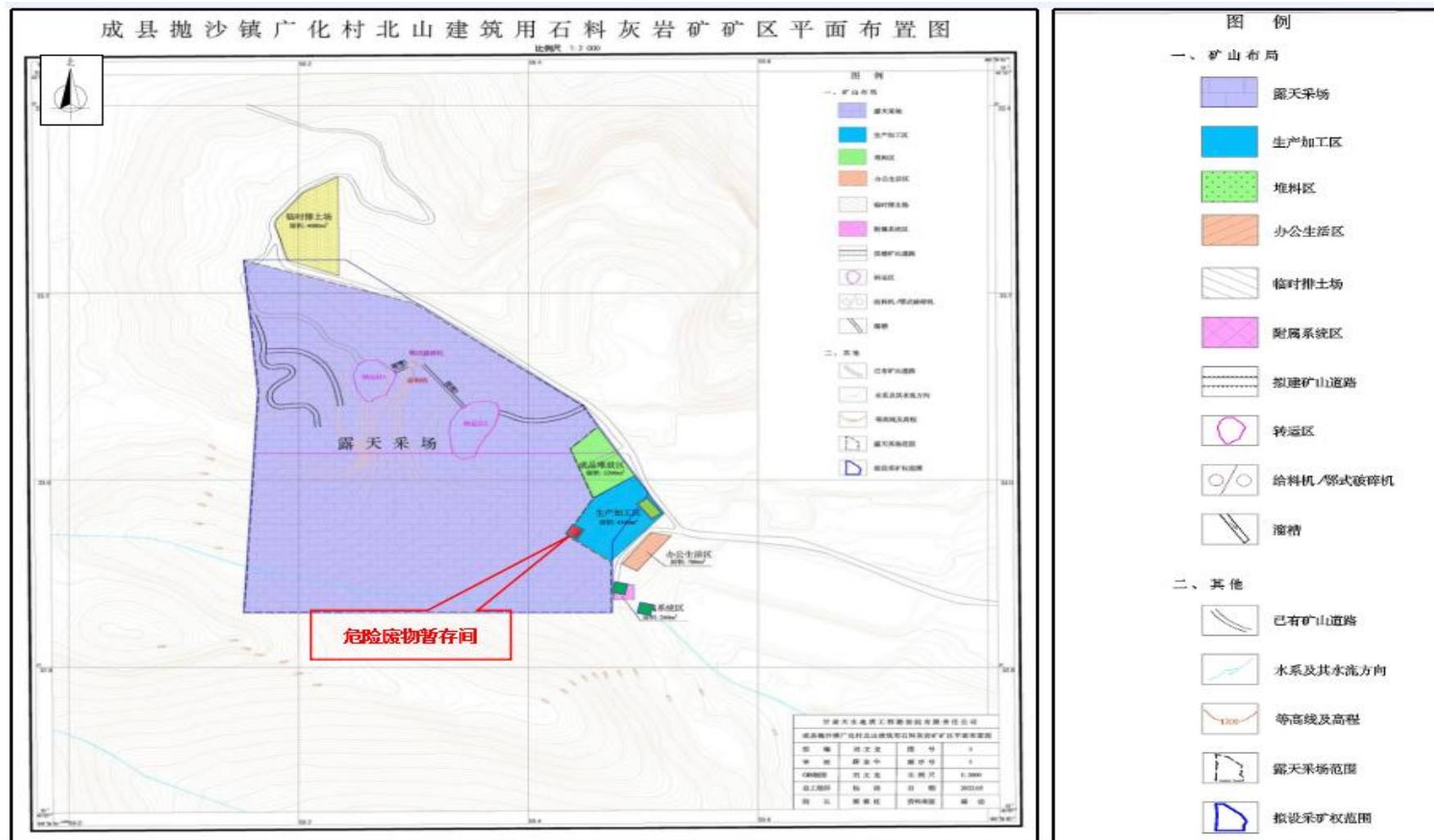
图 2 项目矿区平面布置图
