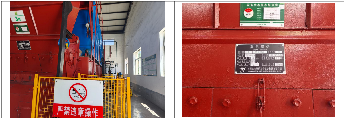
3 号 12t/h 蒸汽锅炉（生产供蒸汽）
